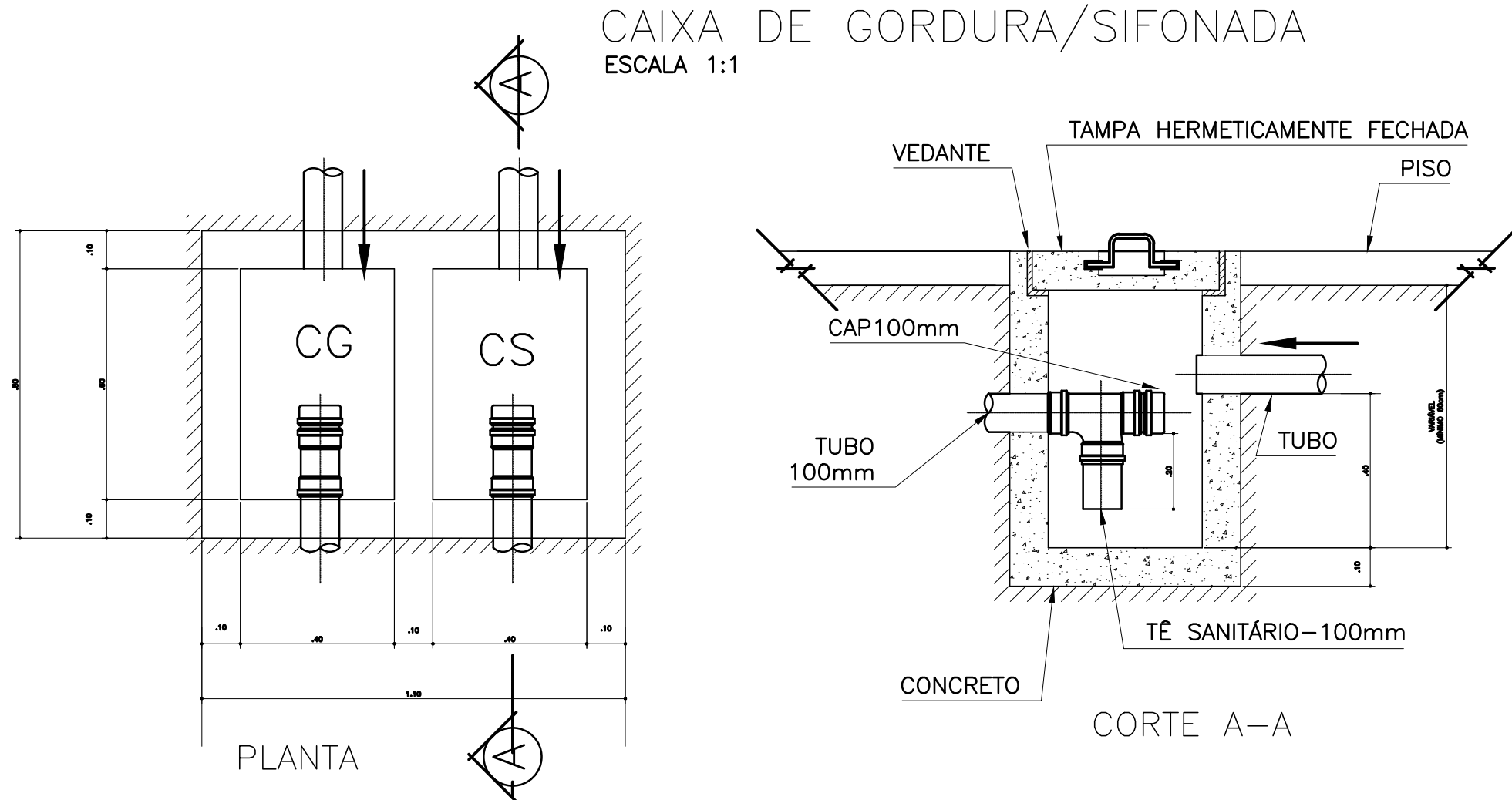
DETALHE CAIXA DE GORDURA ESC. 1:50
