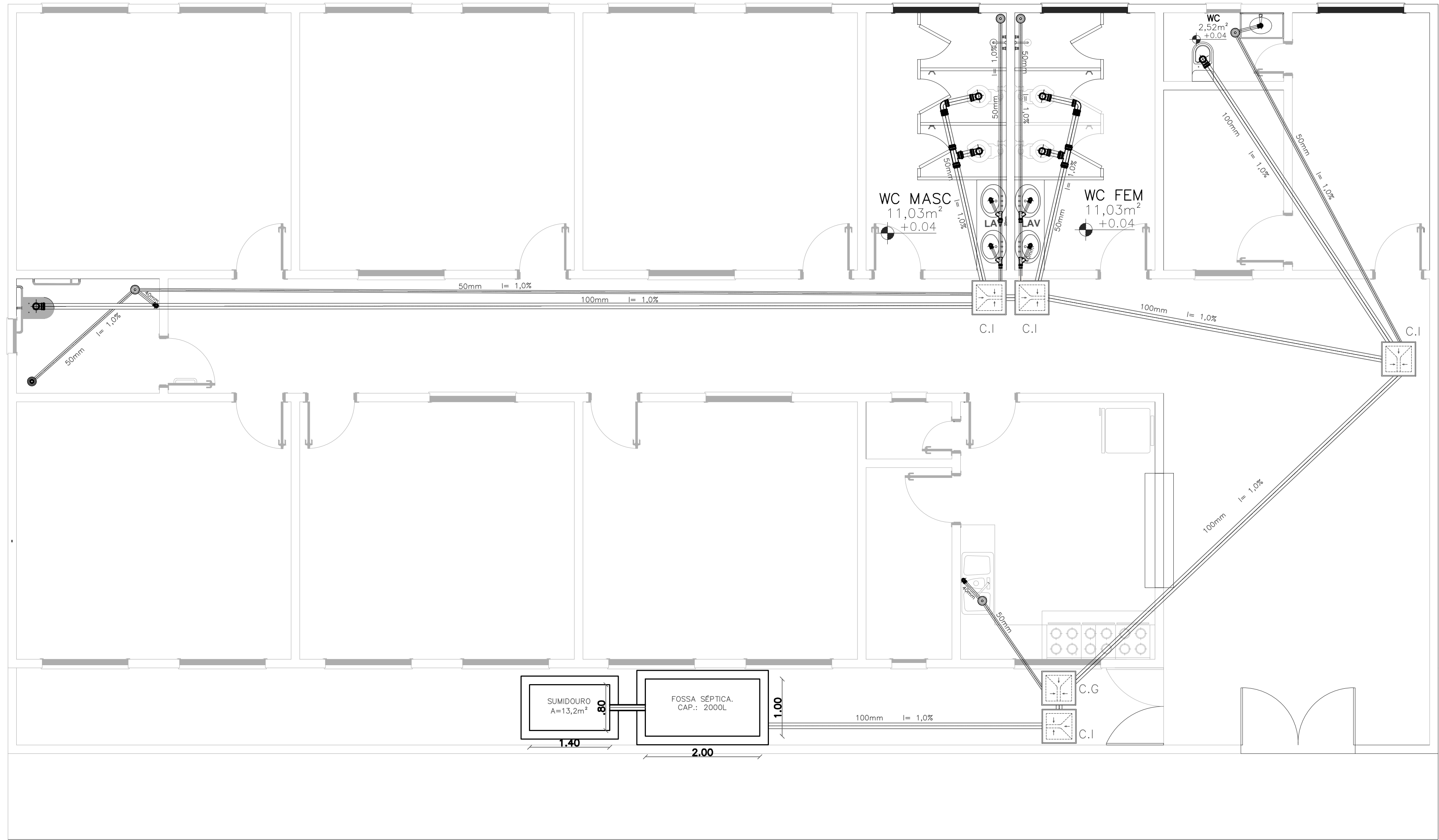
PROJETO HIDROSSANITÁRIO EMEIF PESSOA PIRES ESC. 1:100
