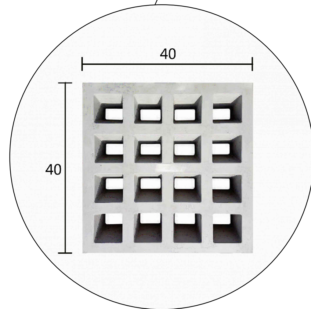
COBOGÓ 16 FUROS ANTI CHUVA ESC. 1:50
