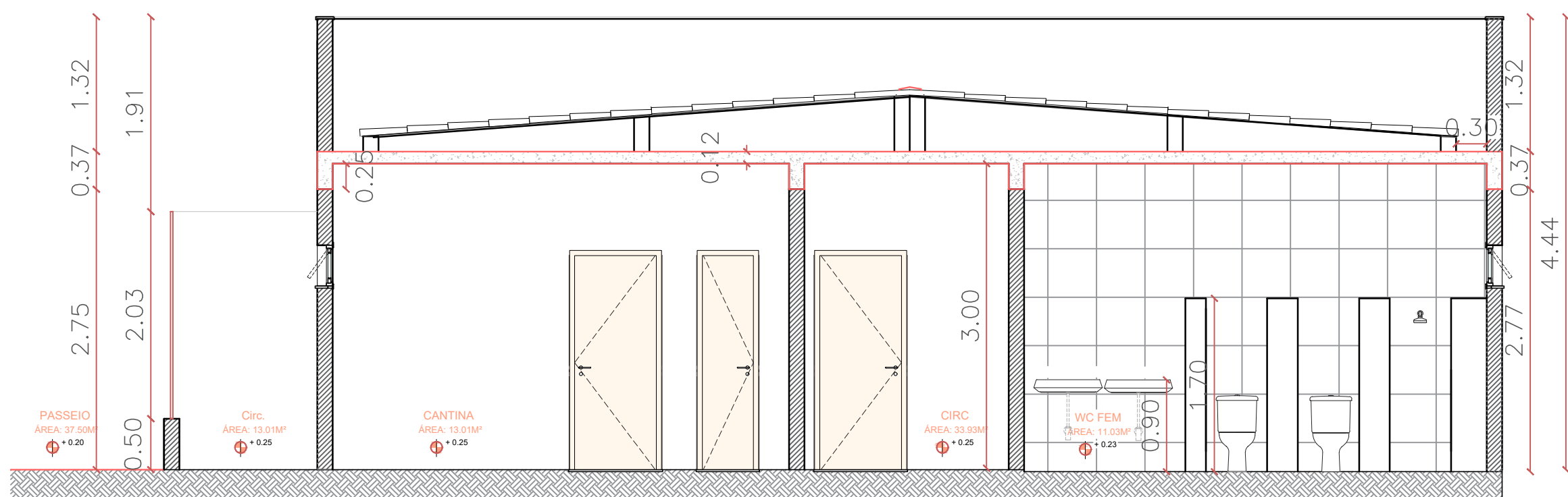
CORTE CC ESC. 1:50
