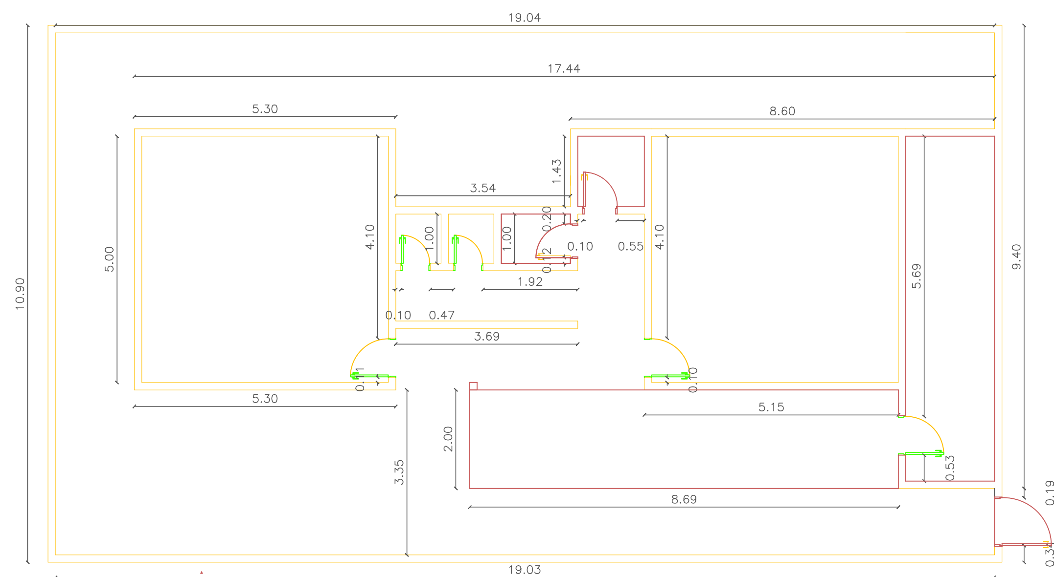
PLANTA BAIXA ATUAL - LEVANTAMENTO ESC. 1:75
