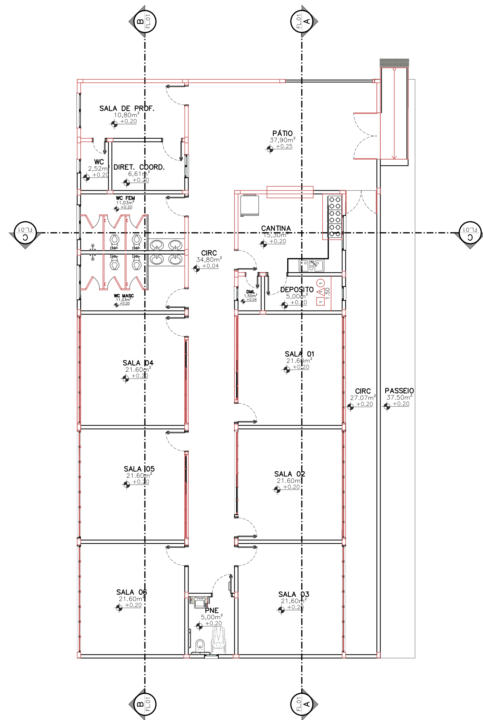
PLANTA DE REFERÊNCIA ESC. 1:100
