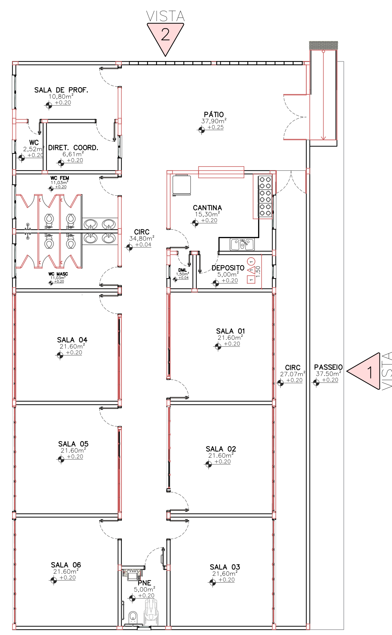
PLANTA DE REFERÊNCIA ESC. 1:100
