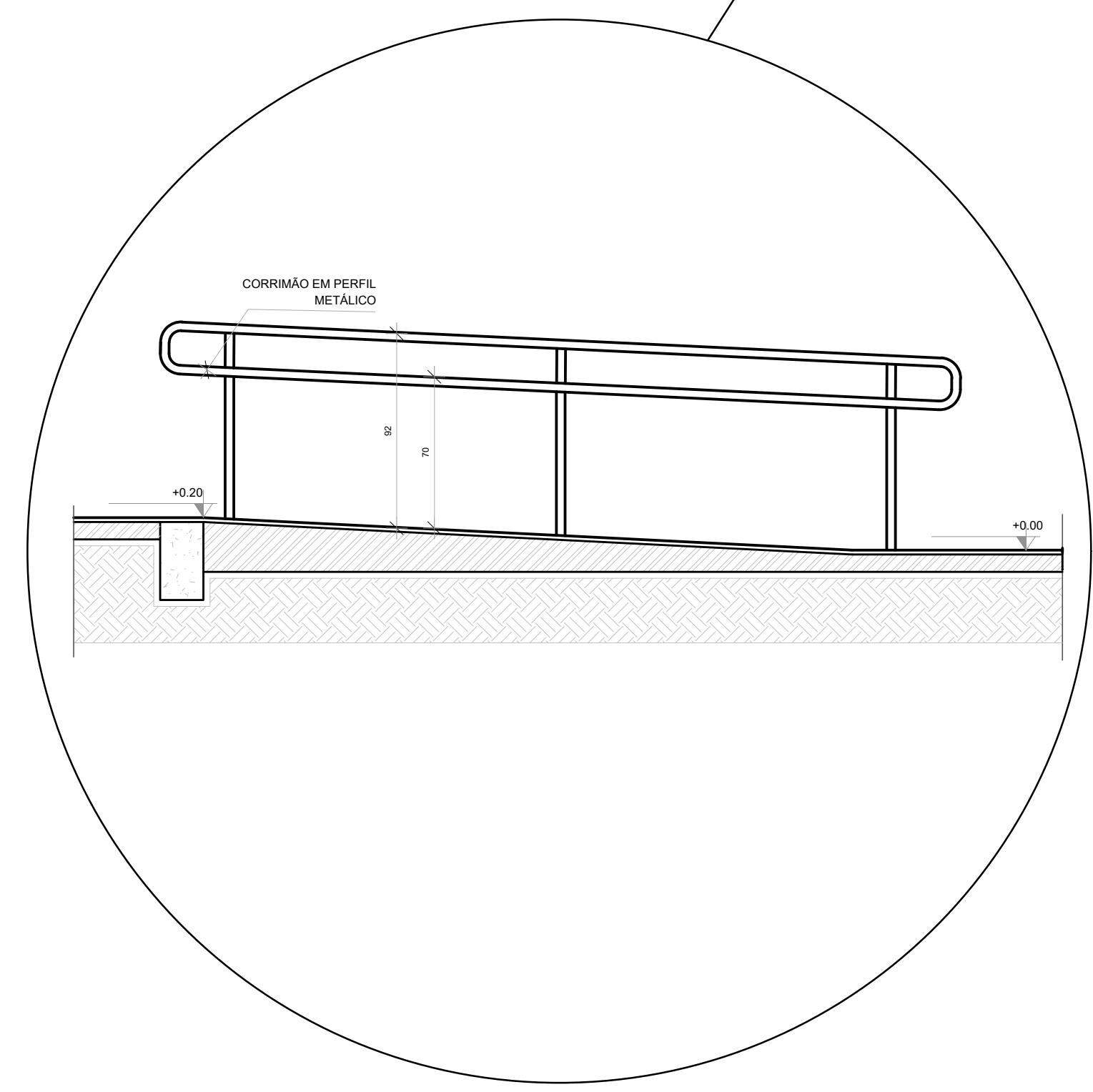
DETALHE RAMPA ESC. 1:50
