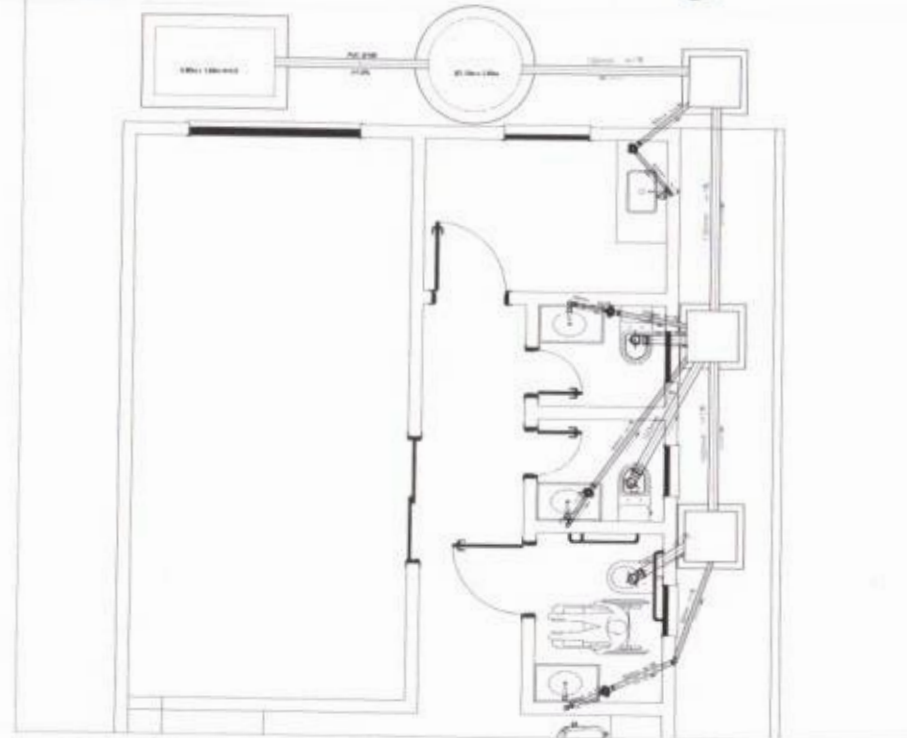
01 DETALHE PROJETO SANITÁRIO
