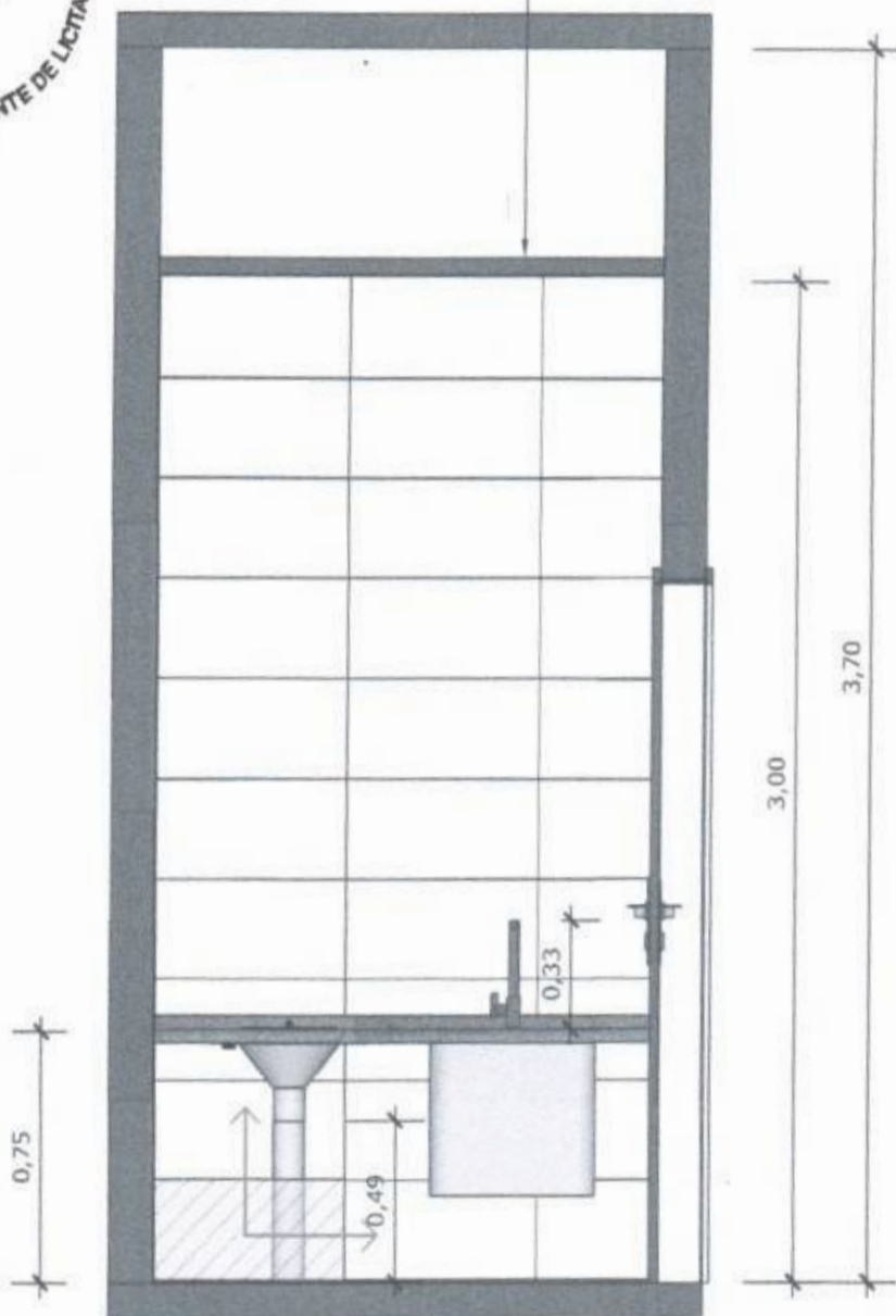
28 VISTA 01 Escala: 1/25
