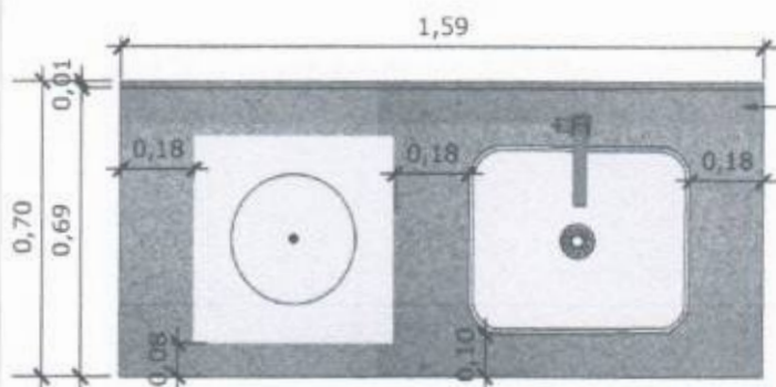
29 VISTA SUPERIOR BANCADA
