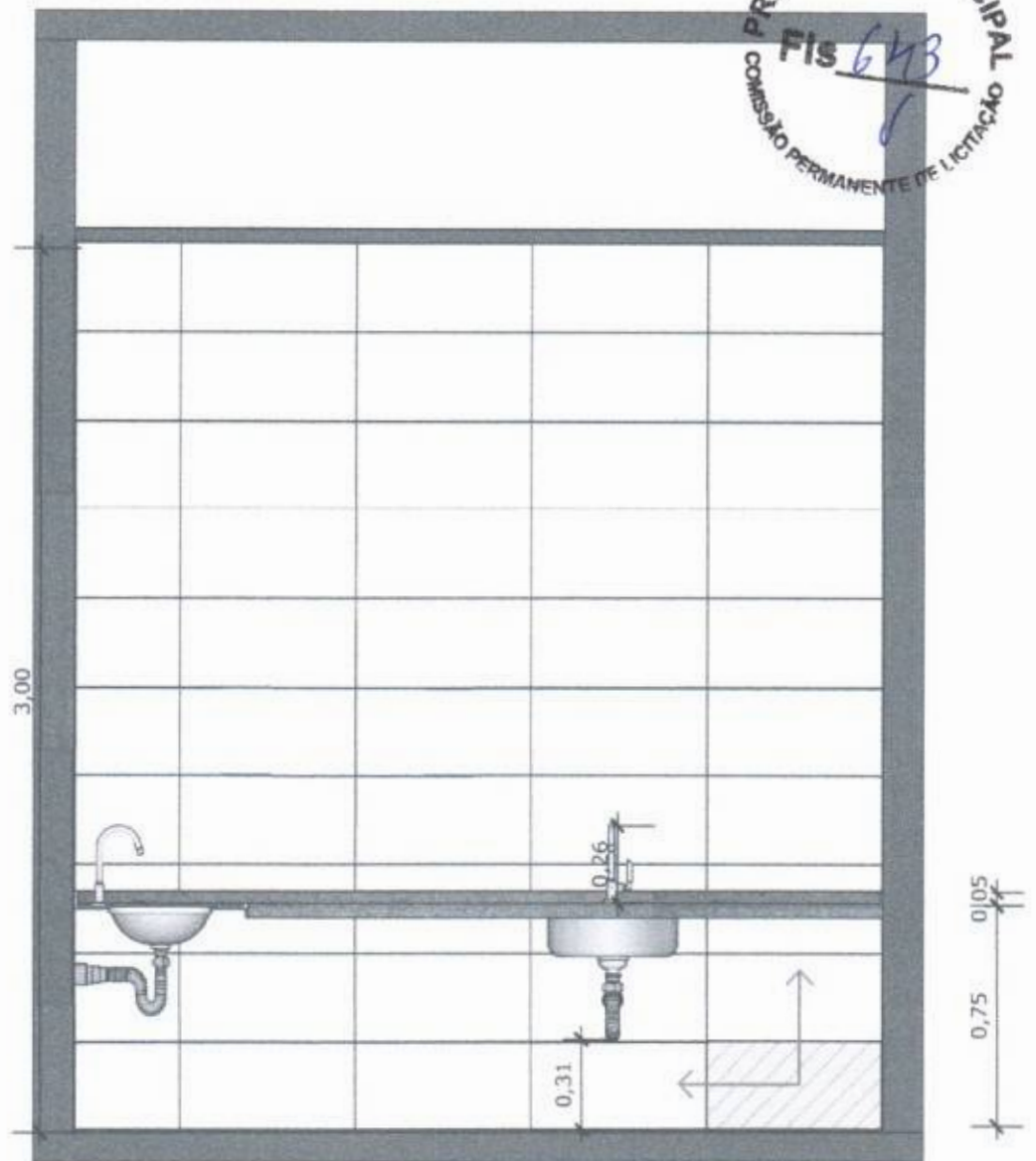
36 VISTA 01 Escala: 1/25
