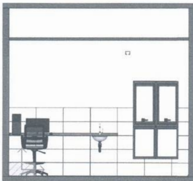
77 VISTA 01 Escala: 1/50
