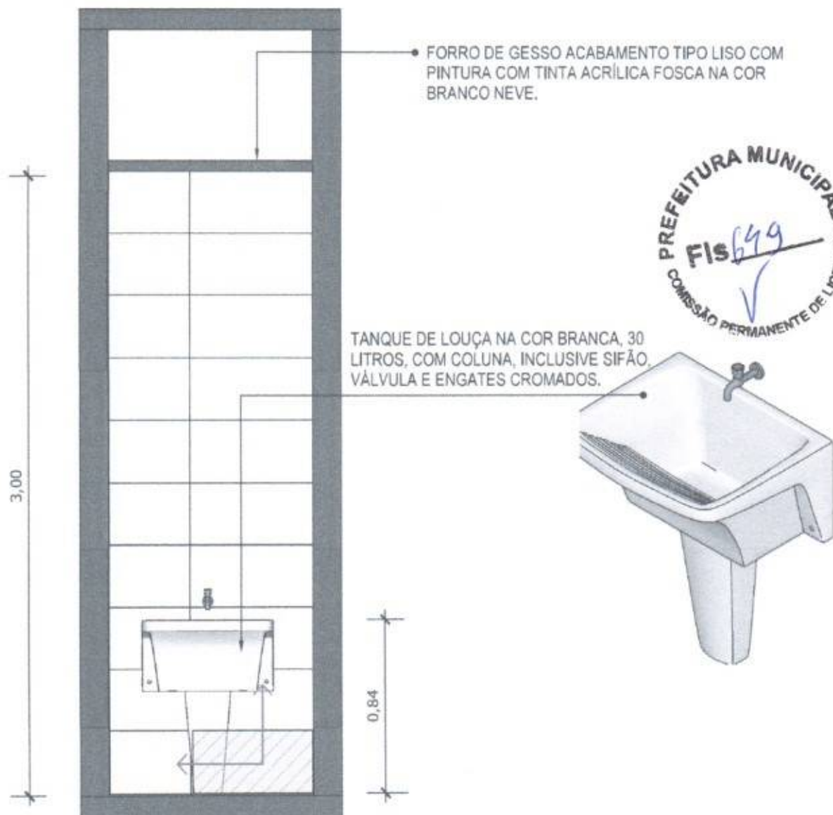
45 VISTA 01 Escala: 1/25
