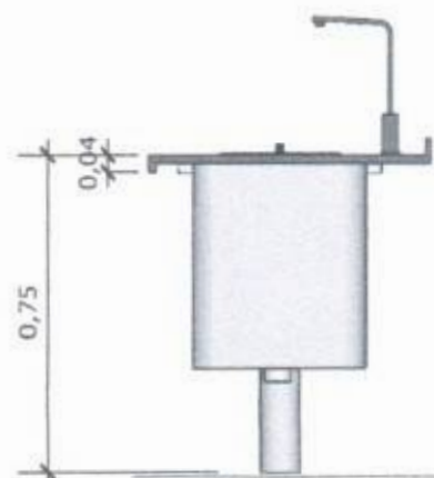
32 VISTA FRONTAL BANCADA
