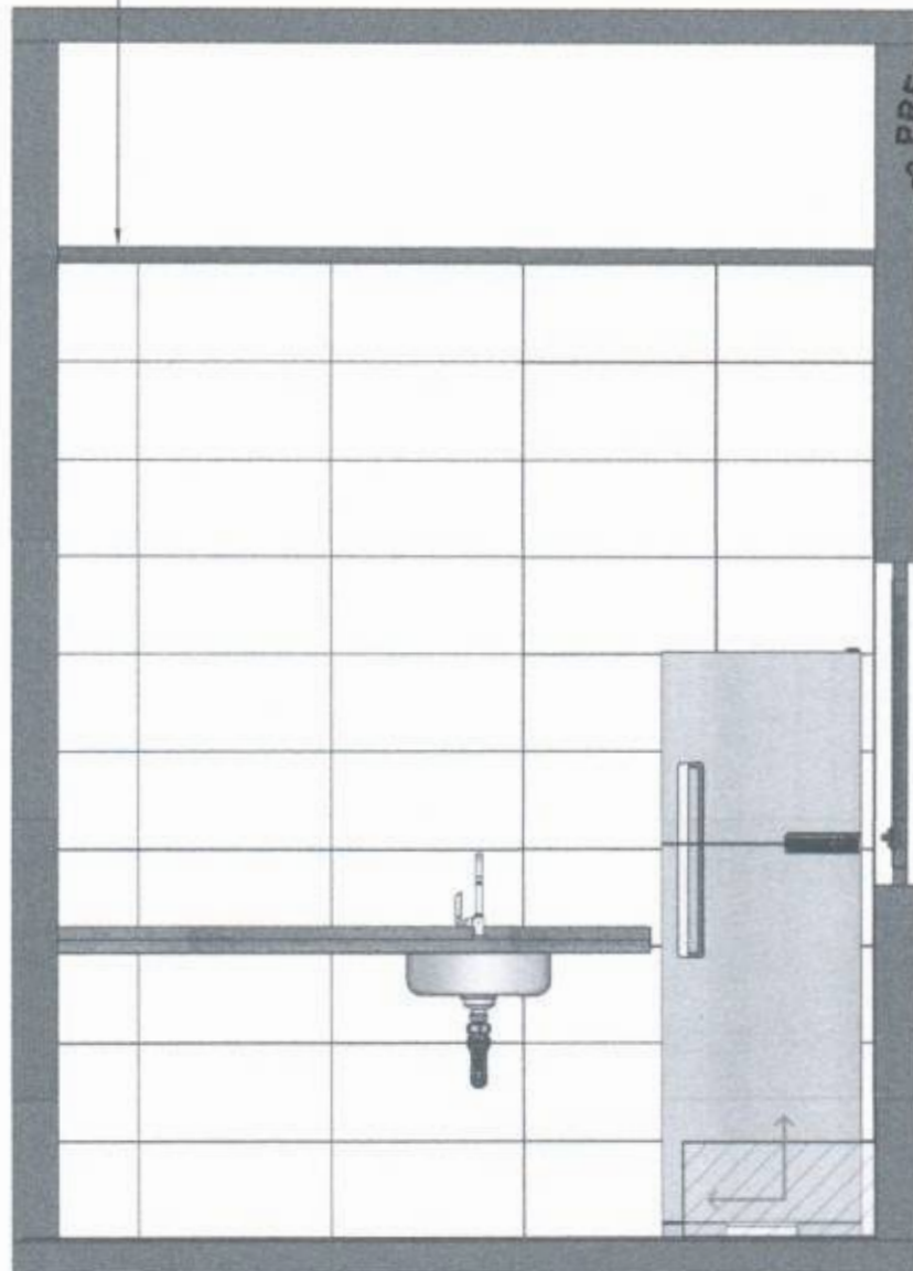
49 VISTA 01 Escala: 1/25
