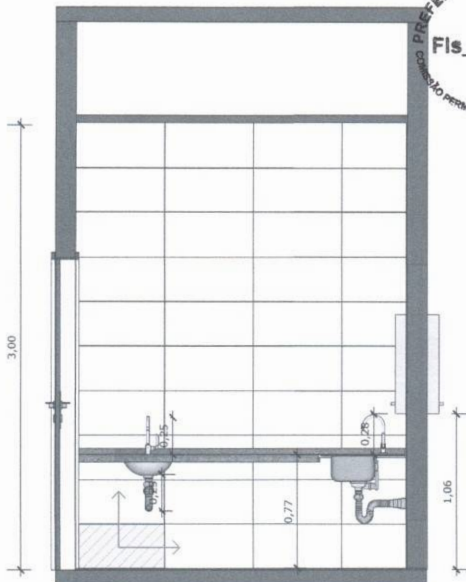
37 VISTA 02 Escala: 1/25
