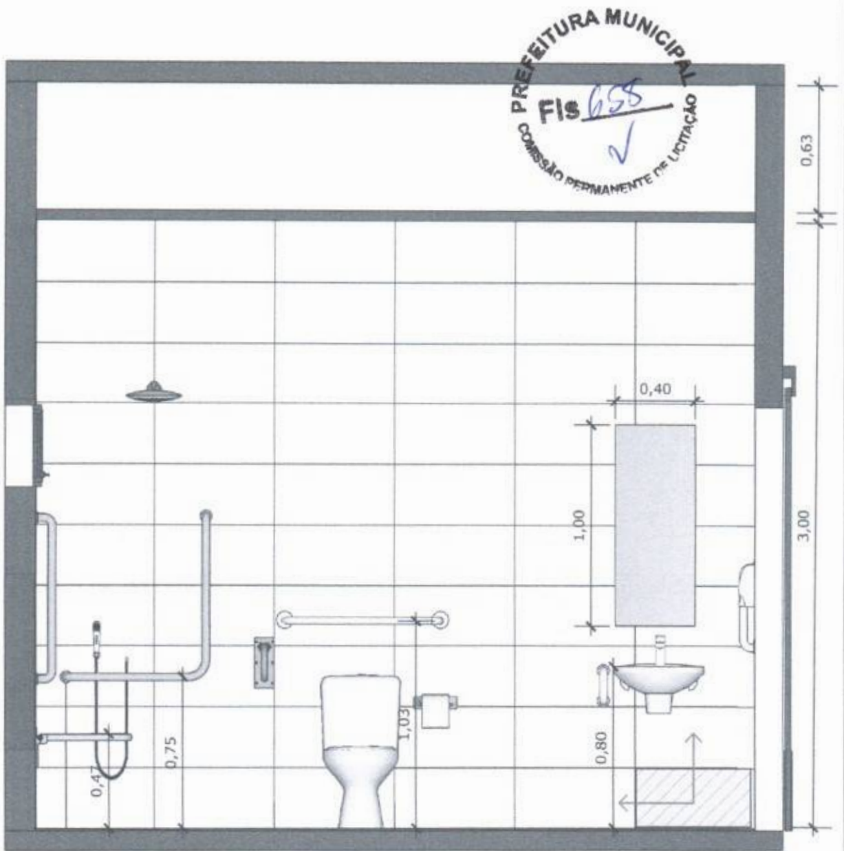
57 VISTA 01 Escala: 1/25
