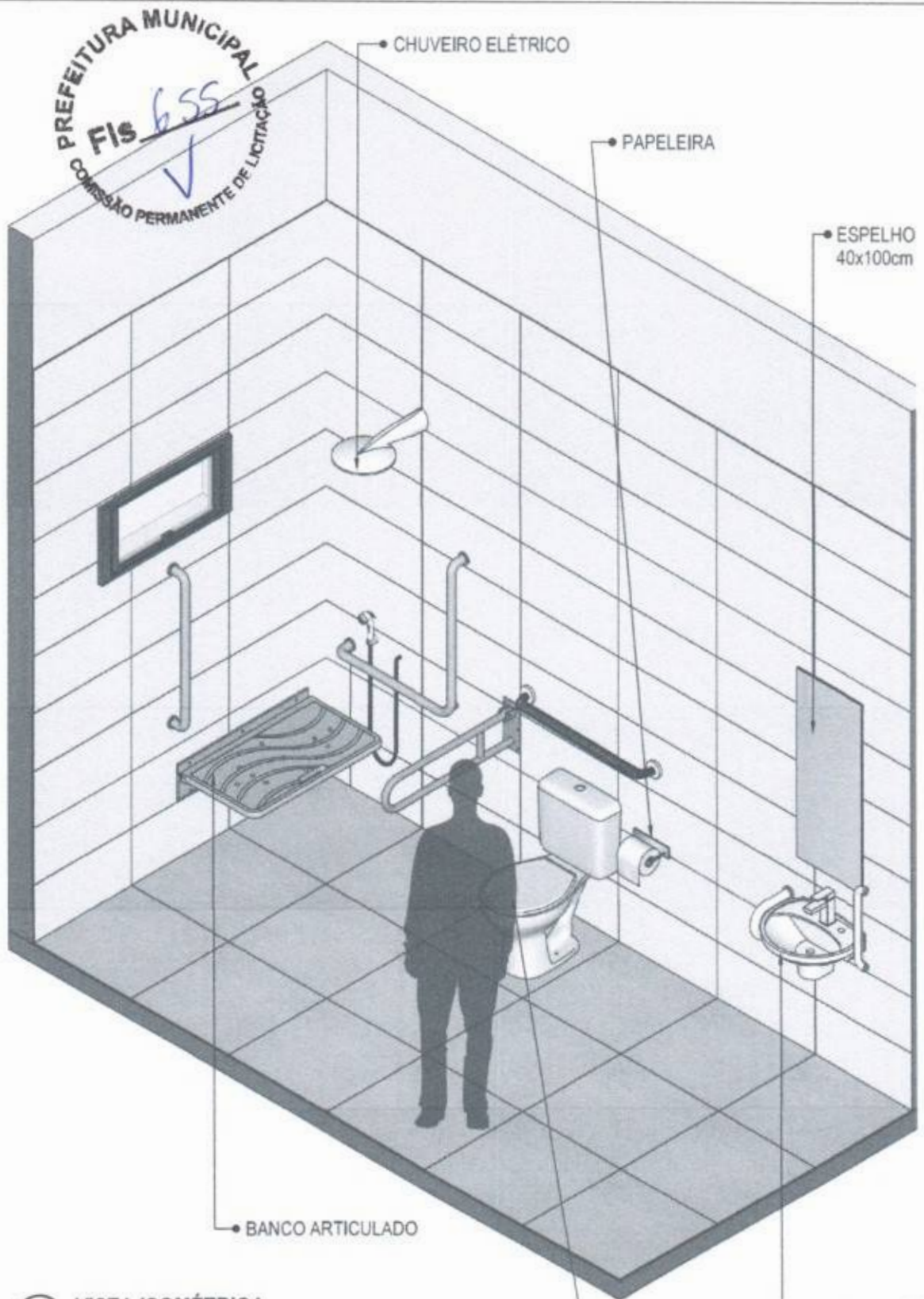
54 VISTA ISOMÉTRICA Escala: 1/25
