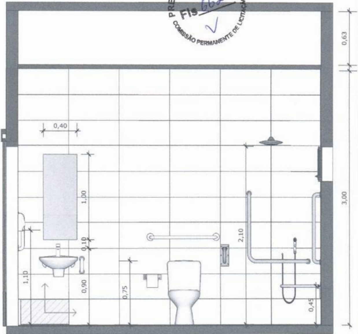
61 VISTA 01 Escala: 1/25
