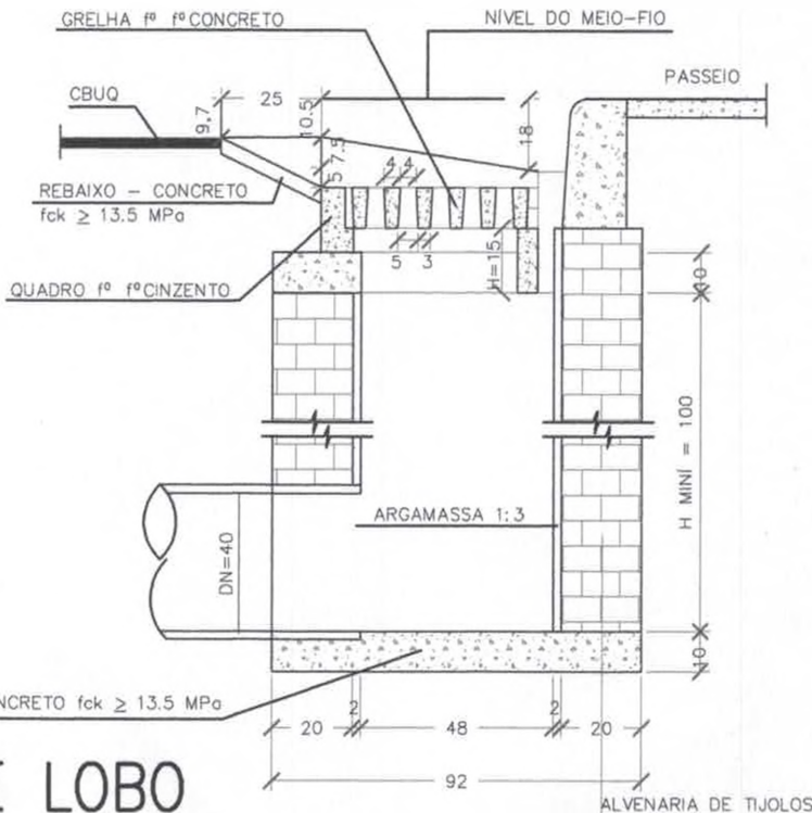
CORTE B-B ESC. SEM ESCALA
