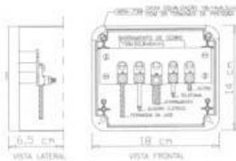
BASE DE IGUALIZAÇÃO DOS POTENCIAIS 18x14mm EM PVC DETALHE SEM ESCALA
