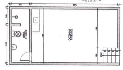
02 SUBSOLO - COZINHA escala 1/20
